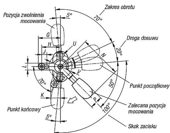
Wykonanie prawostronne
