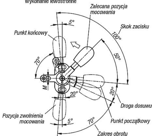
Wykonanie lewostronne
