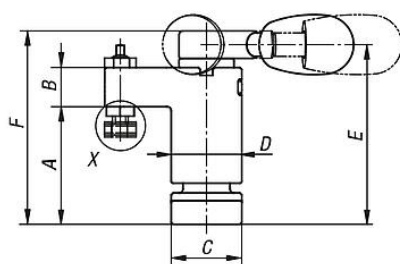
Wykonanie prawostronne
