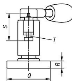
Wykonanie lewostronne
