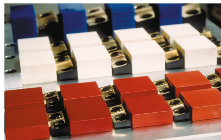
Przykład rozwiązania przyrządu wielogniazdowego z użyciem kostek dociskowych bocznych
