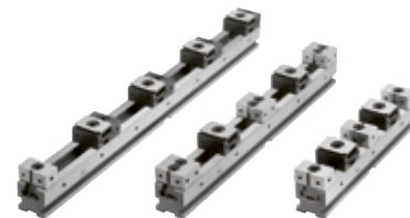
Vícenásobný upínací systém
