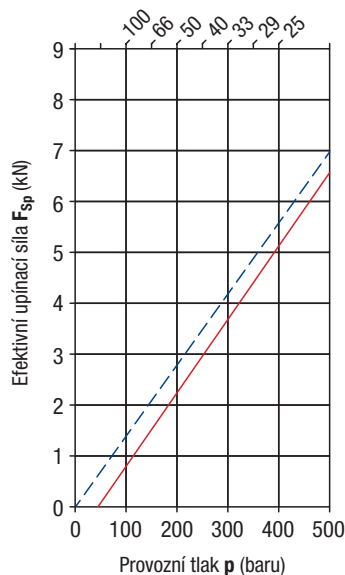
Píst-Ø 25 mm
