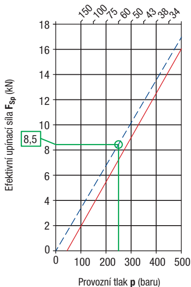
Píst-Ø 40 mm
