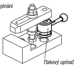
Horizontální upínání
