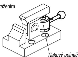
Vertikální upínání
