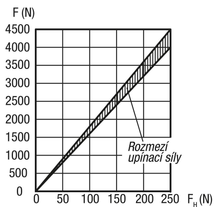
Silový diagram
